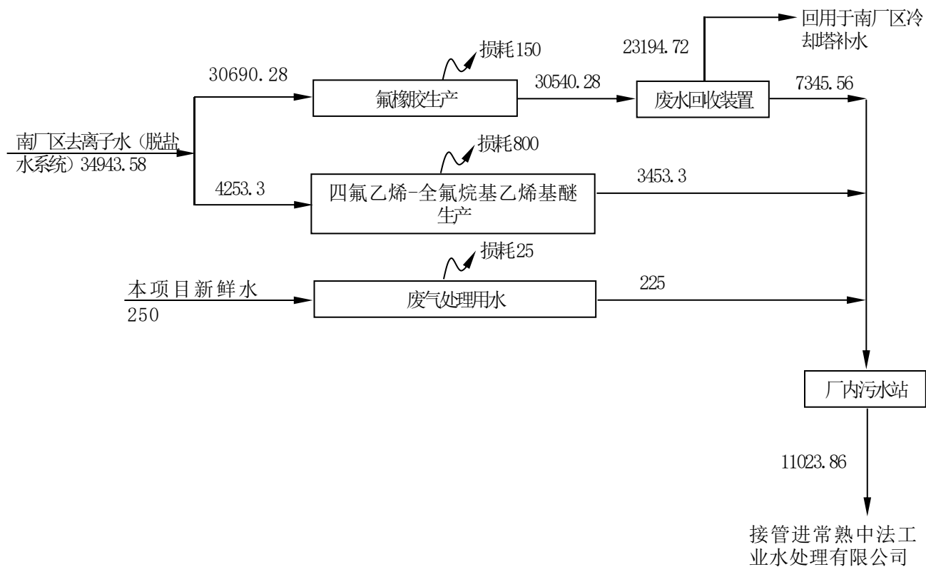
图 4.7-2 本项目水平衡图 (m³/a)
