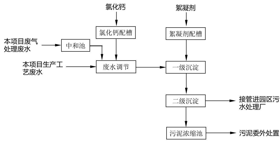
图 7.2-2 厂区污水站处理工艺流程
