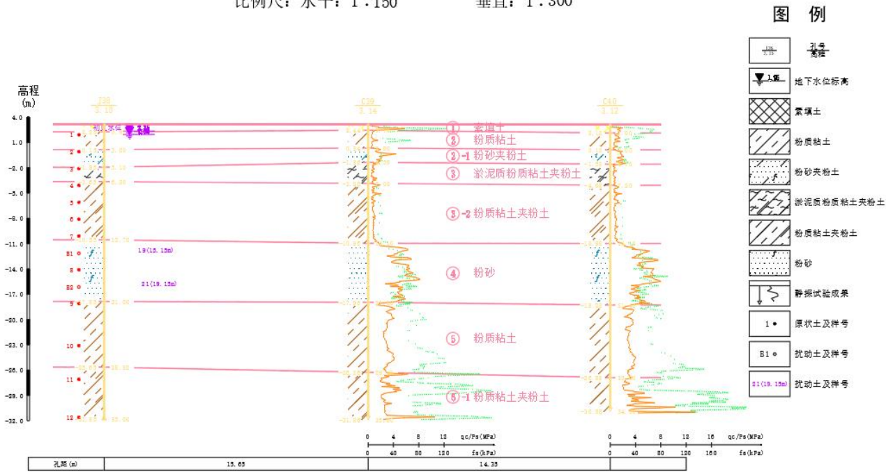
图 6.5.1.1 场地典型地质剖面图
