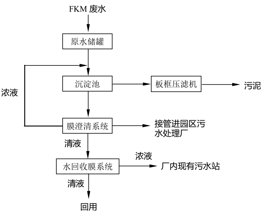
图 7.2-1 氟橡胶废水回用装置工艺流程图
