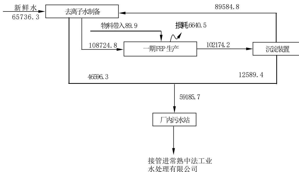
图 3.7 1000t/a 聚全氟乙丙烯水平衡图
