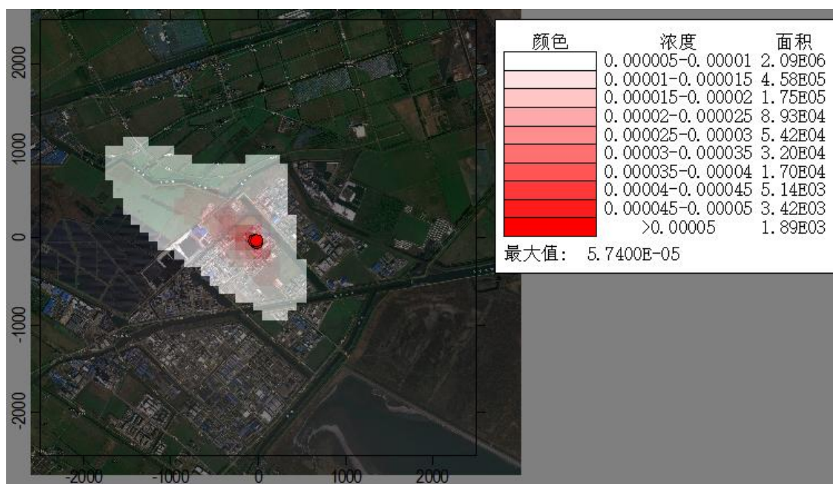
图 6.1.5-4 颗粒物年均最大浓度贡献值等值线分布图
