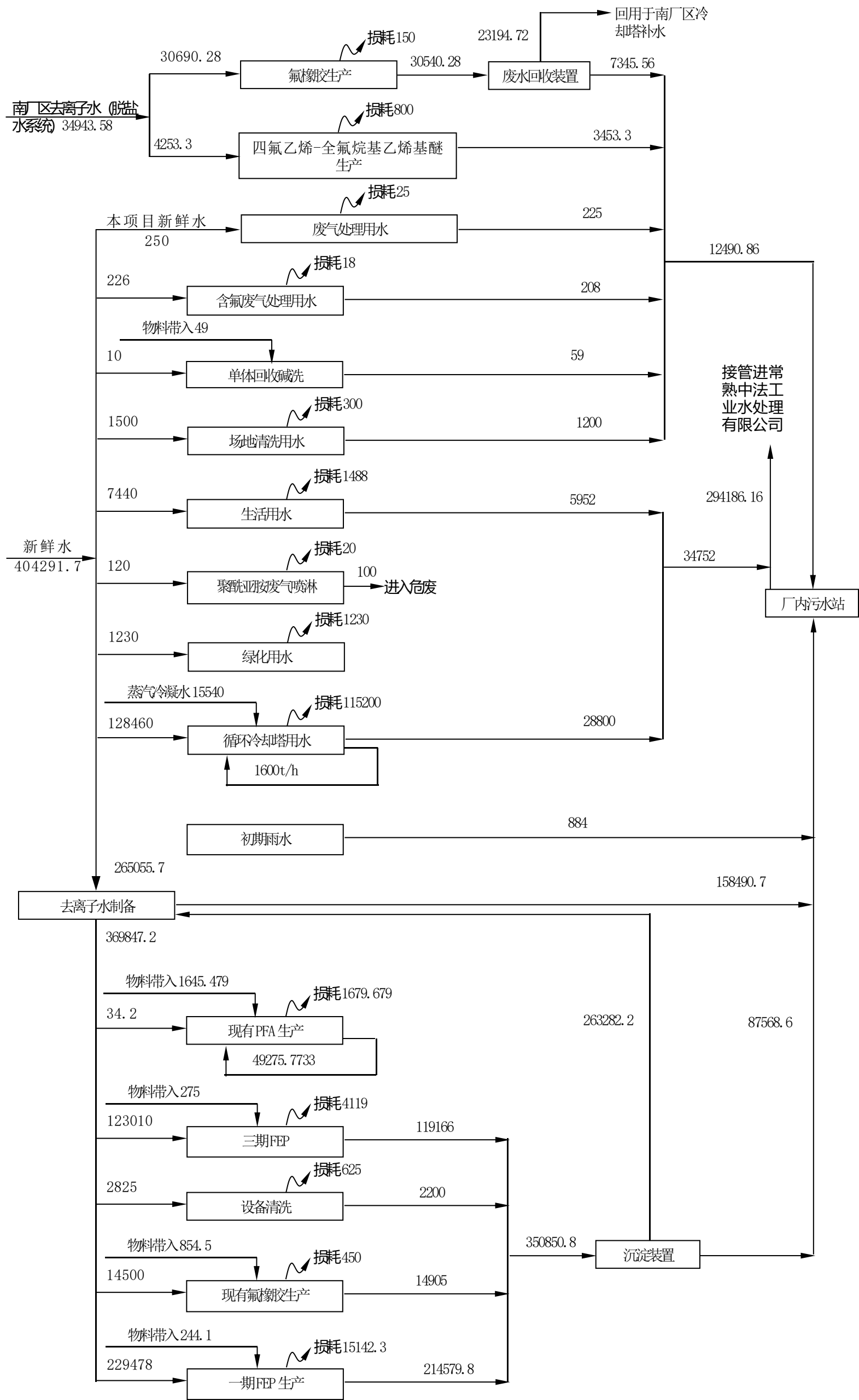
图 4.7-3 本项目建成后全厂水平衡图 (m³/a)
