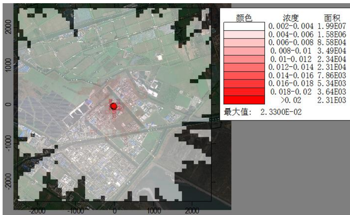
图 6.1.5-1 非甲烷总烃小时最大浓度贡献值等值线分布图
