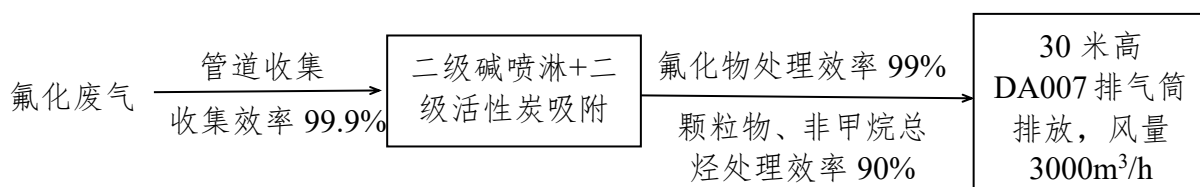
图 7.1.1-1 本项目废气处理工艺流程图
