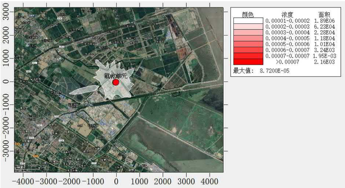
图 6.2.1-8 PM 2.5 小时最大浓度贡献值等值线分布图
