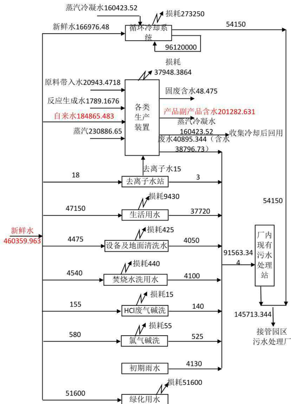
图 3.4.2-2 技改后全厂水平衡图 (单位: t/a)
