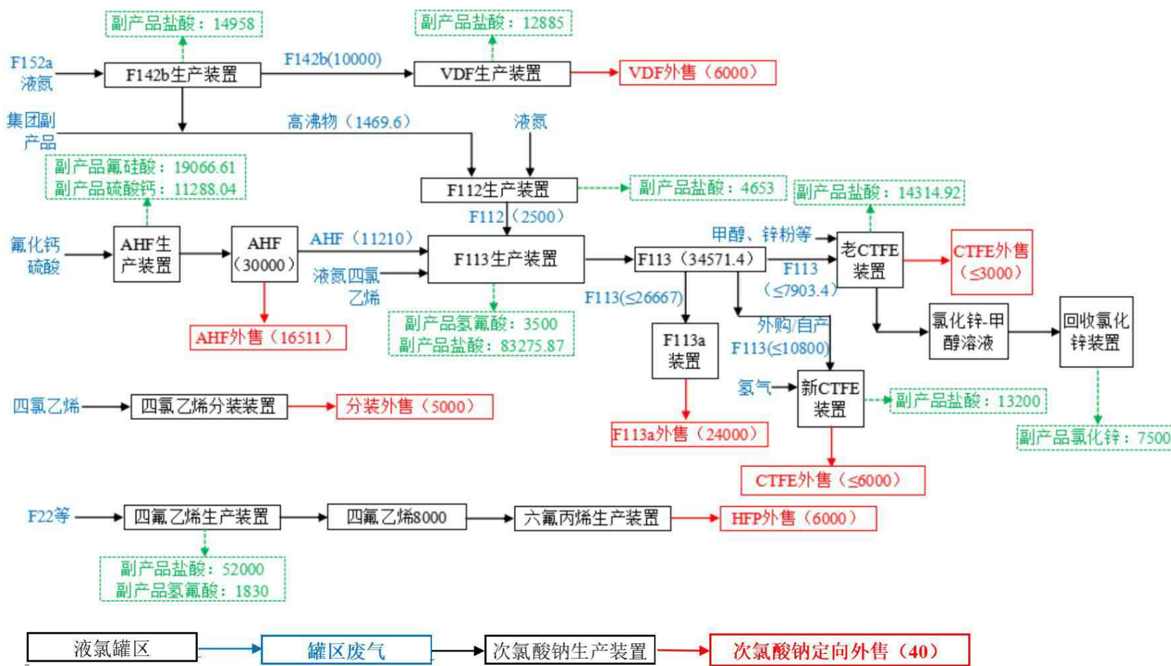
图 3.2.2-1 拟建项目完成后三爱富公司全厂产品链示意图 (单位: t/a)
