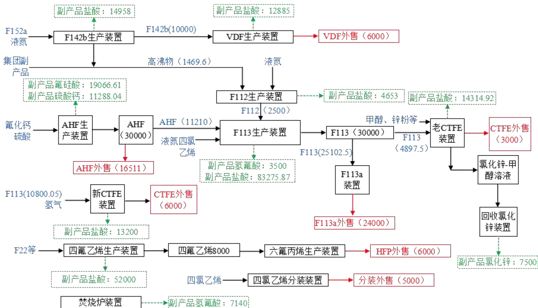
图 3.1.1-1 三爱富公司现有项目产品链示意图（单位：t/a）
