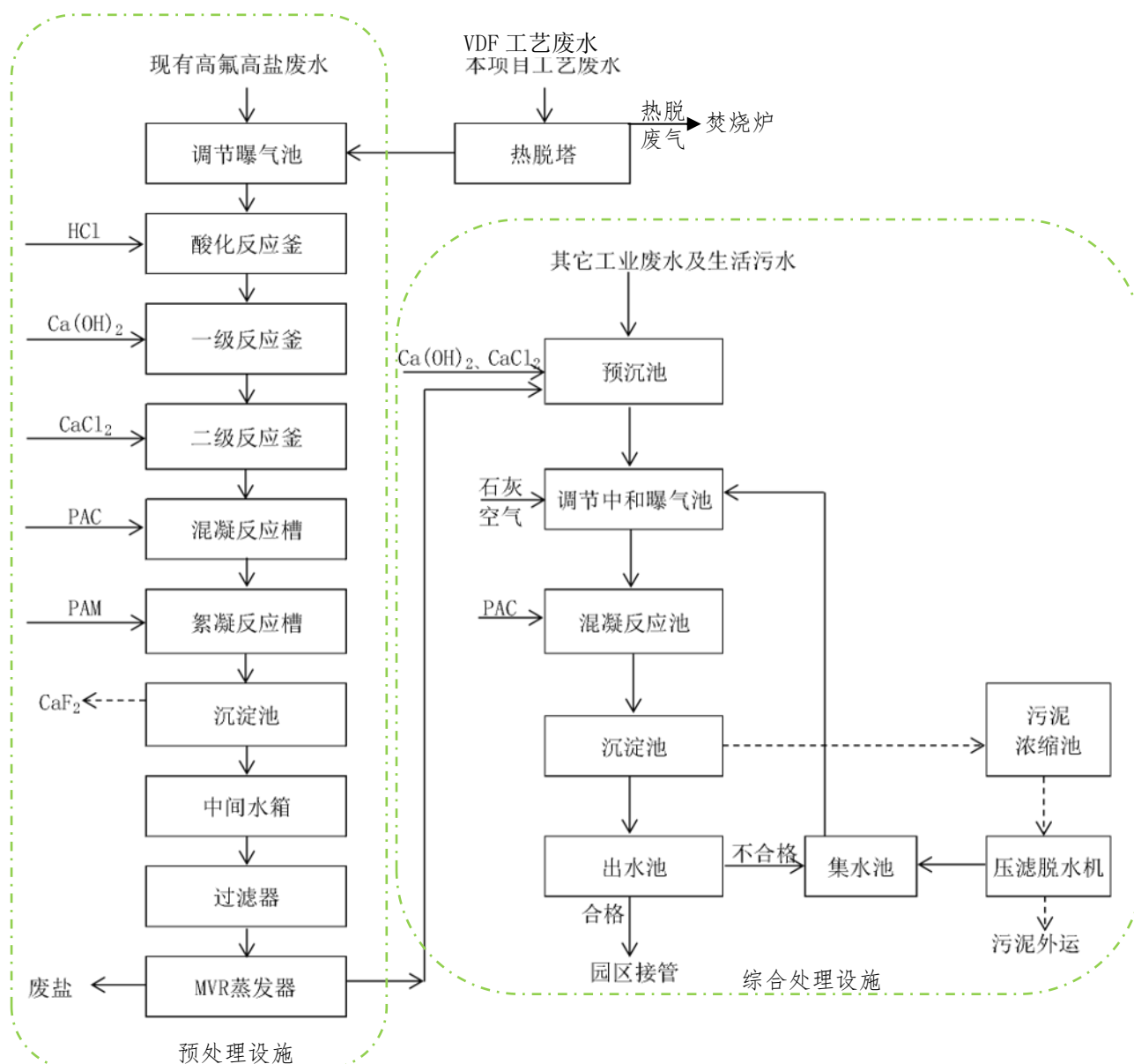
3.1.5-1 污水处理站工艺流程图
