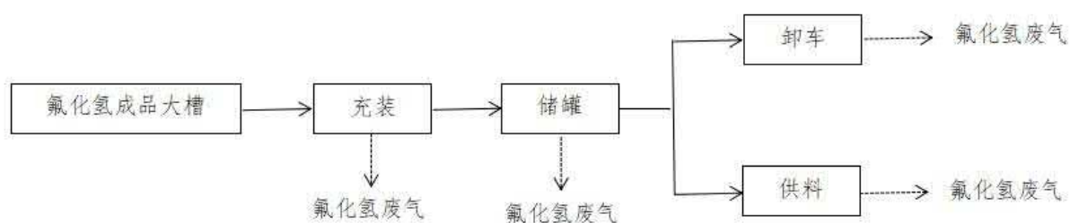
图 3.3.2-2 氟化氢储罐装卸工艺流程及产污环节图
