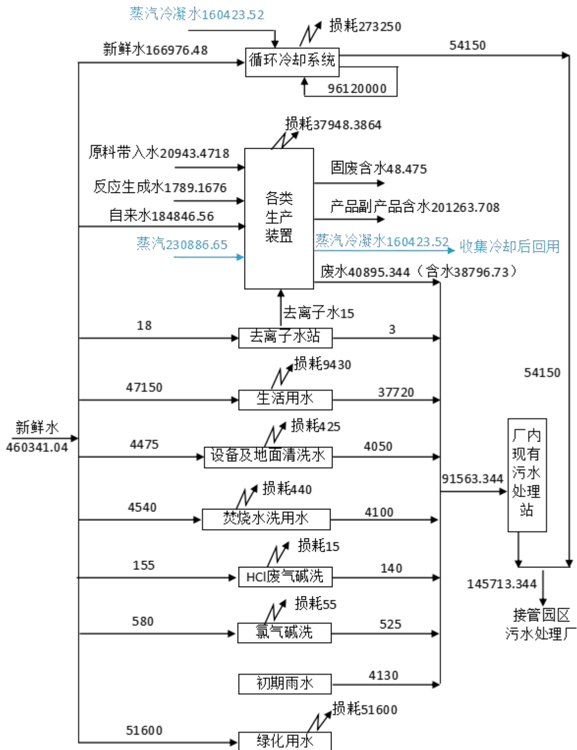
图 3.1.4-1 现有项目（含在建）全厂水平衡（单位:t/a）
