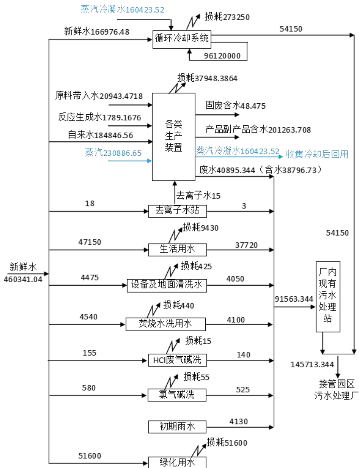
图 3.1.6-1 现有项目（含已批待建+未批待建）全厂水平衡（单位:t/a）
