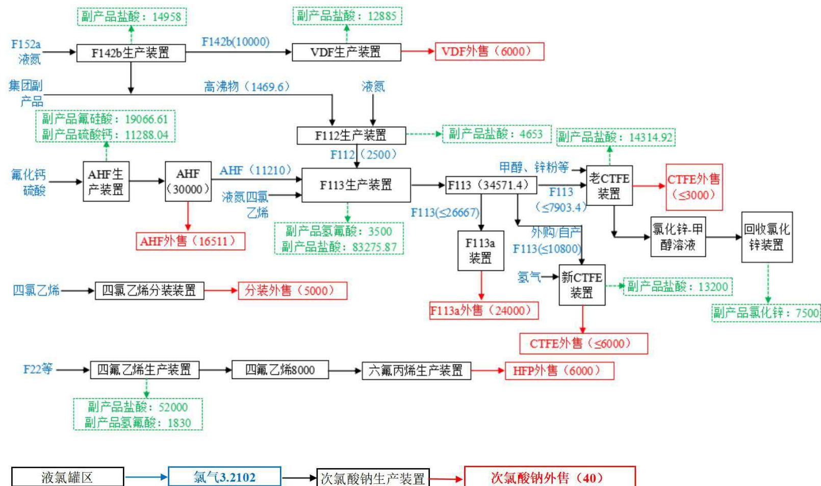
图 3.2.2-1 拟建项目完成后三爱富公司全厂产品链示意图 (单位: t/a)
