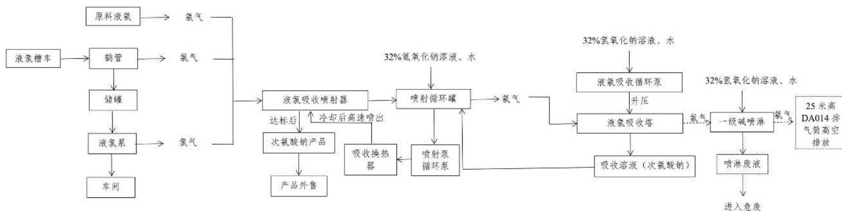
图 3.3.2-1 液氯储罐装卸及次氯酸钠生产工艺流程及产污环节图
