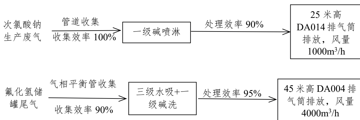
图 6.1-1 本项目废气处理工艺流程图
