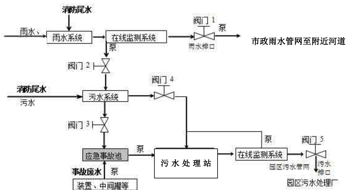
图 6.6.1-2 防止事故废水进入外环境的控制、封堵系统示意图
