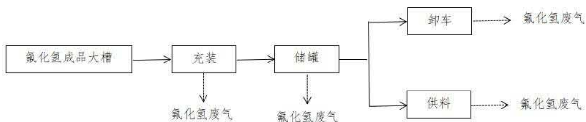
图 3.3.2-3 氟化氢储罐装卸工艺流程及产污环节图 氟化氢储罐装卸工艺流程说明：
