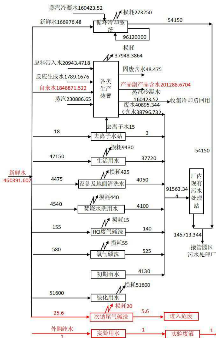
图 3.4.2-2 技改后全厂水平衡图 (单位: t/a)
