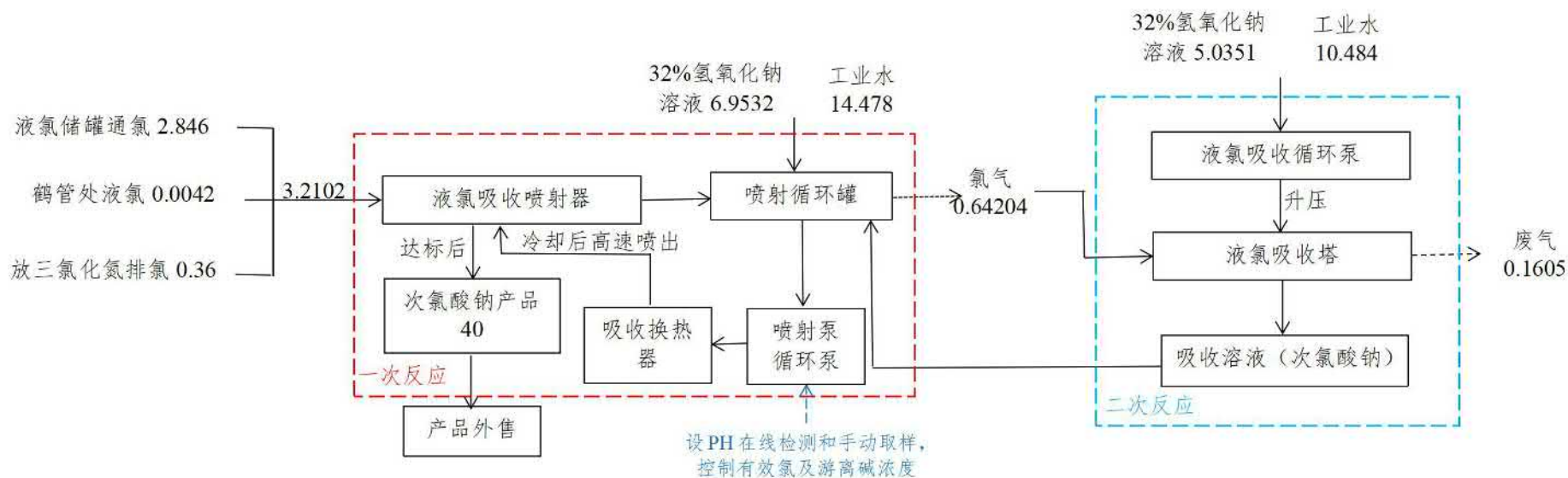
图 3.3.2-2 次氯酸钠生产详细工艺流程图（单位：t/a）
