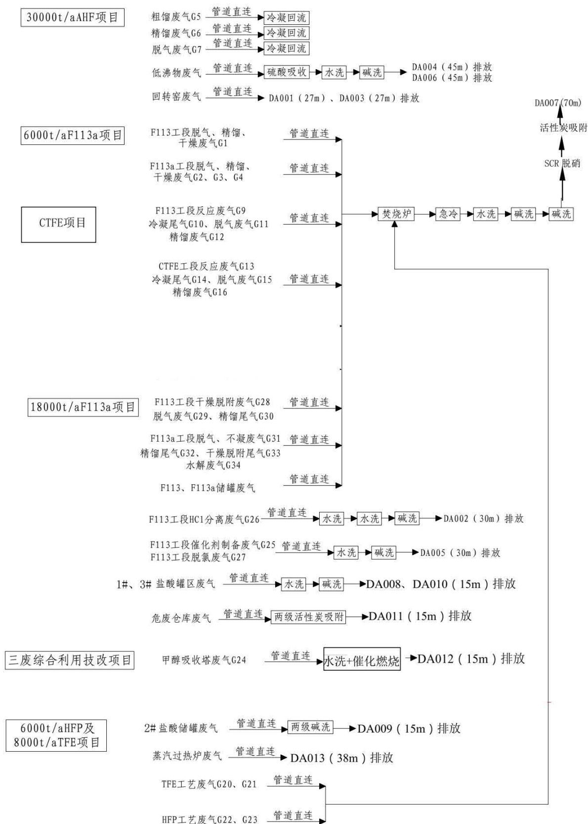
图 3.1.7-2 现有项目废气收集、处理、排放示意图
