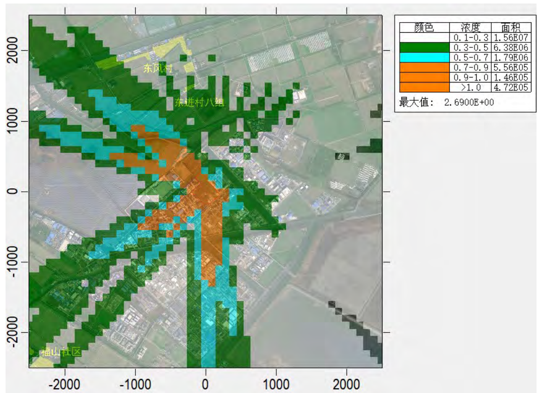
图6.2-21 HCl 1 小时平均质量浓度贡献分布图（单位： \mu\text{g}/\text{m}^3 ）
