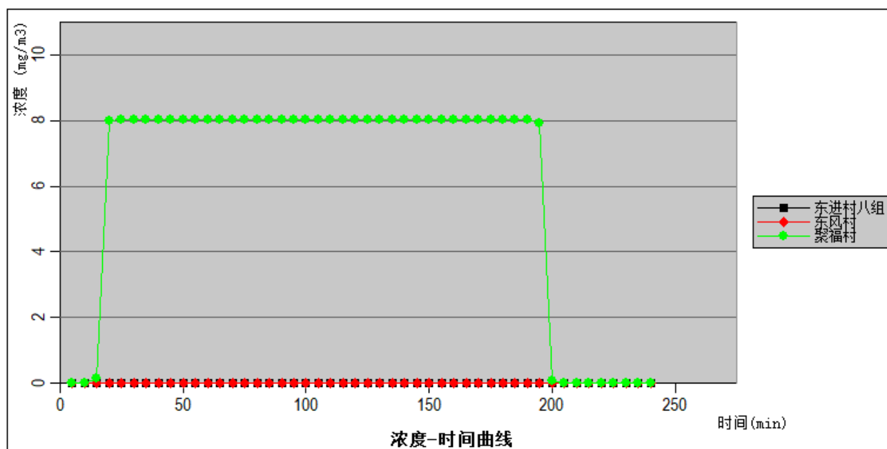
图6.8-31 火灾次生 HF 各敏感点时间与浓度关系图（最常见气象）
