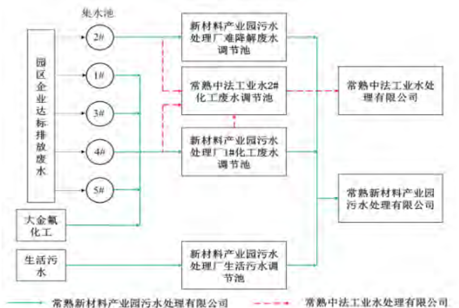
图2.5-1 园区污水收集示意图
