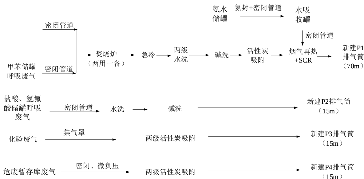
图7.1-1 废气收集及处理示意图
