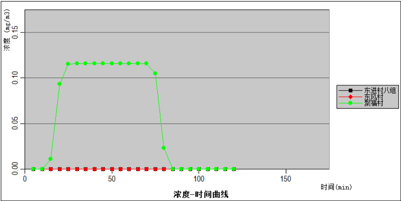
图6.8-16 盐酸（HCl）泄漏各敏感点时间与浓度关系图（最常见气象）
