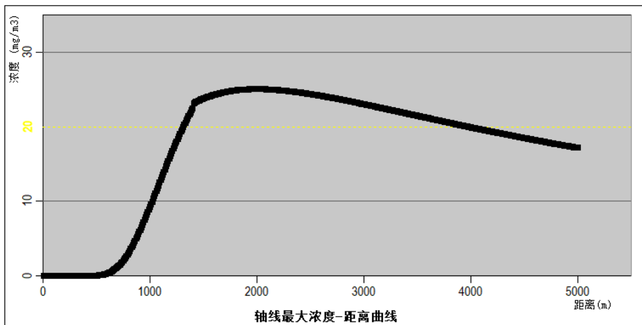
图6.8-28 最不利气象条件下 HF 最大浓度与距离关系图
