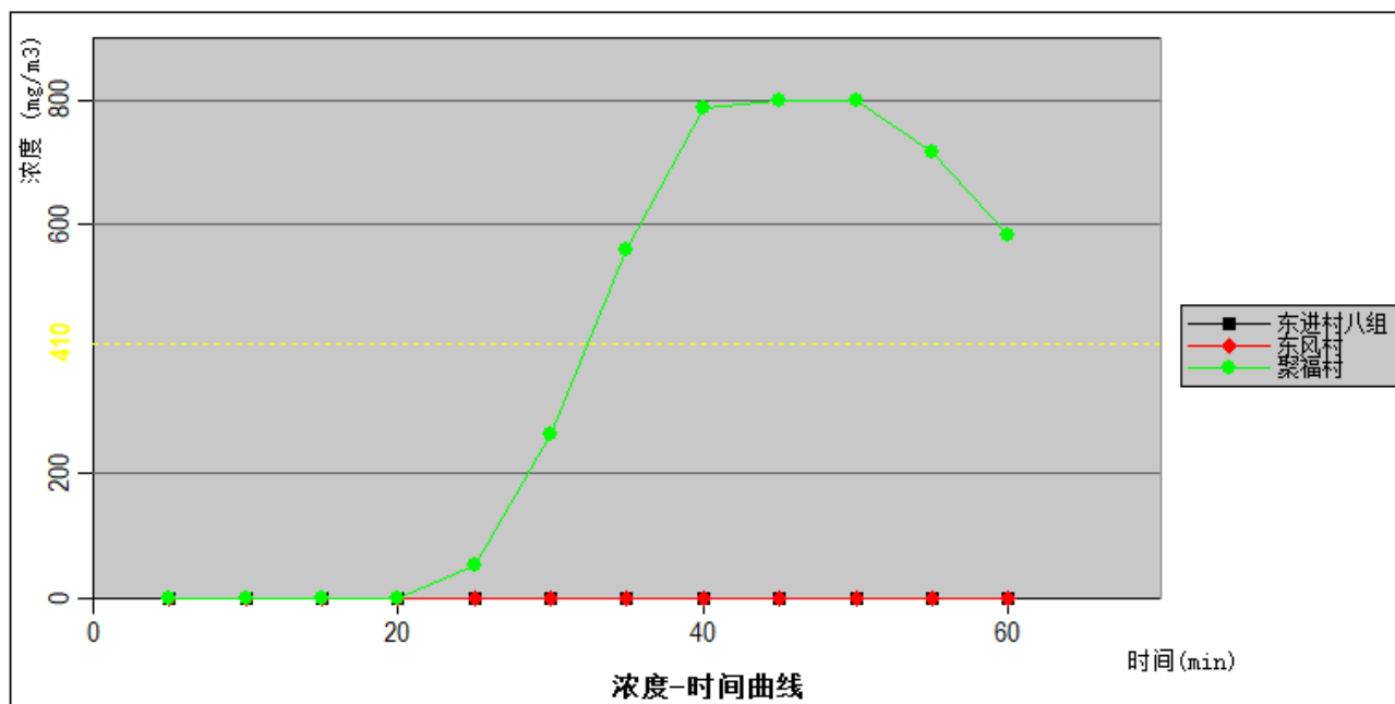
图6.8-5 CTFE 泄漏各敏感点时间与浓度关系图（最不利气象）
