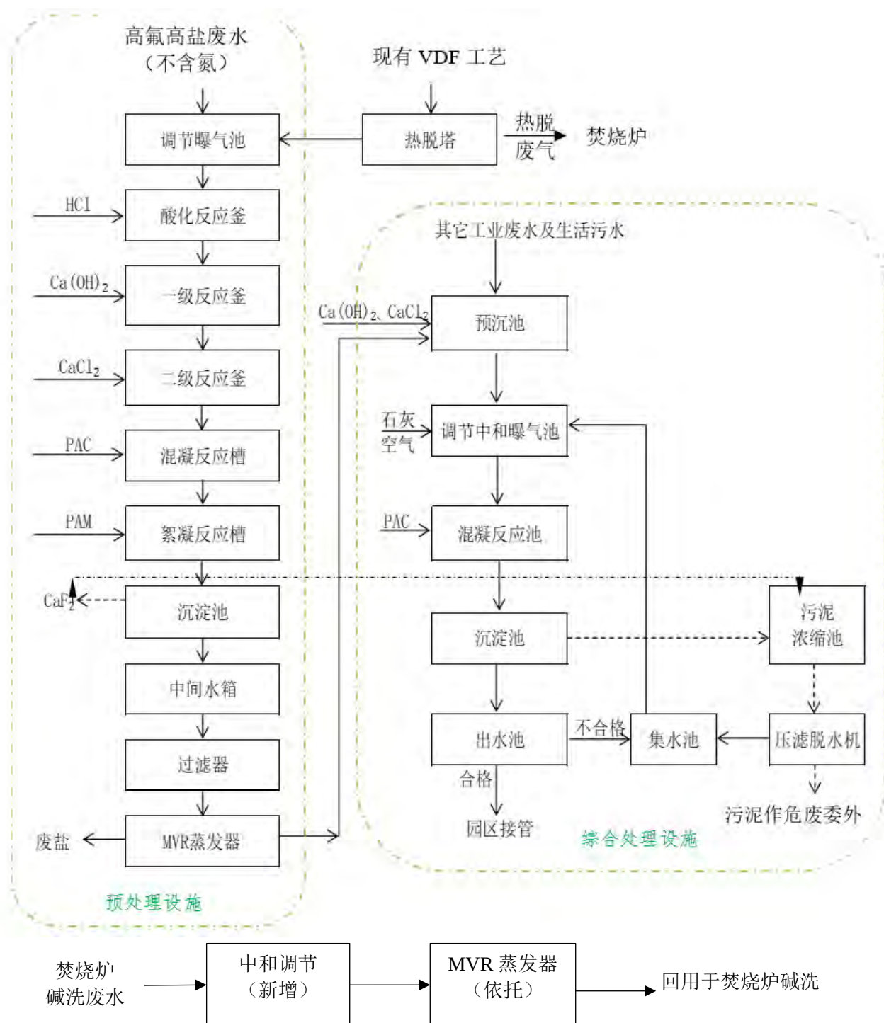
图7.2-1 三爱富公司全厂废水收集及处理系统示意图
