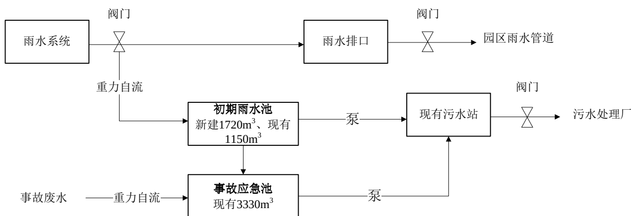
图7.6-1 事故废水防范和处理系统
