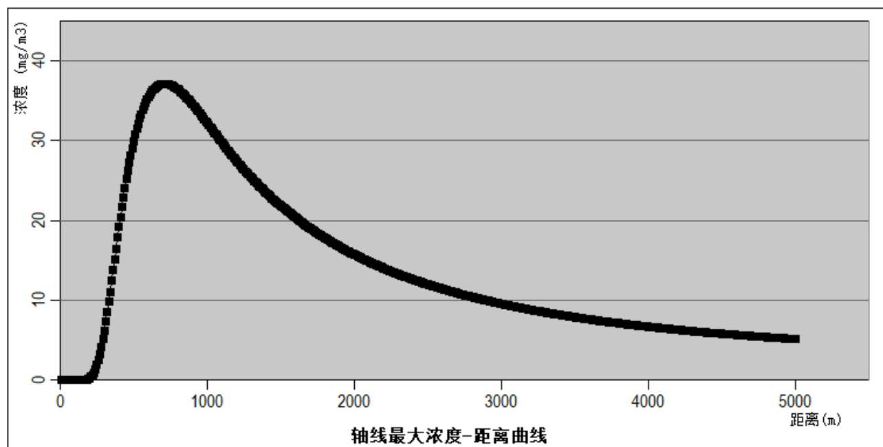
图6.8-33 最常见气象条件下***最大浓度与距离关系图
