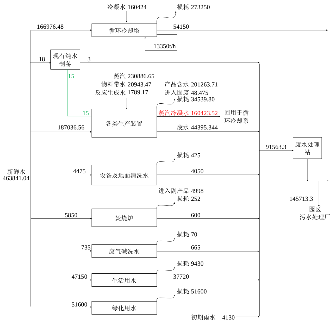
图3.5-1 现有项目（含在建、待建）全厂水平衡（单位：t/a）
