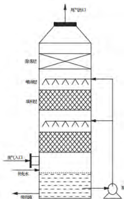
图7.1-3 喷淋吸收工艺示意图
