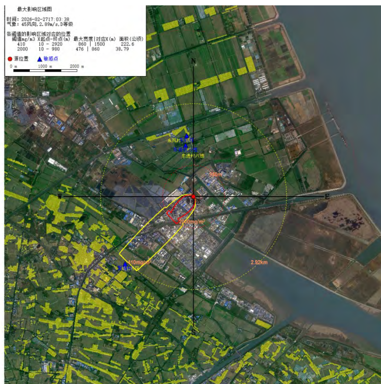
图6.8-2 最常见气象条件下 CTFE 泄漏影响范围图
