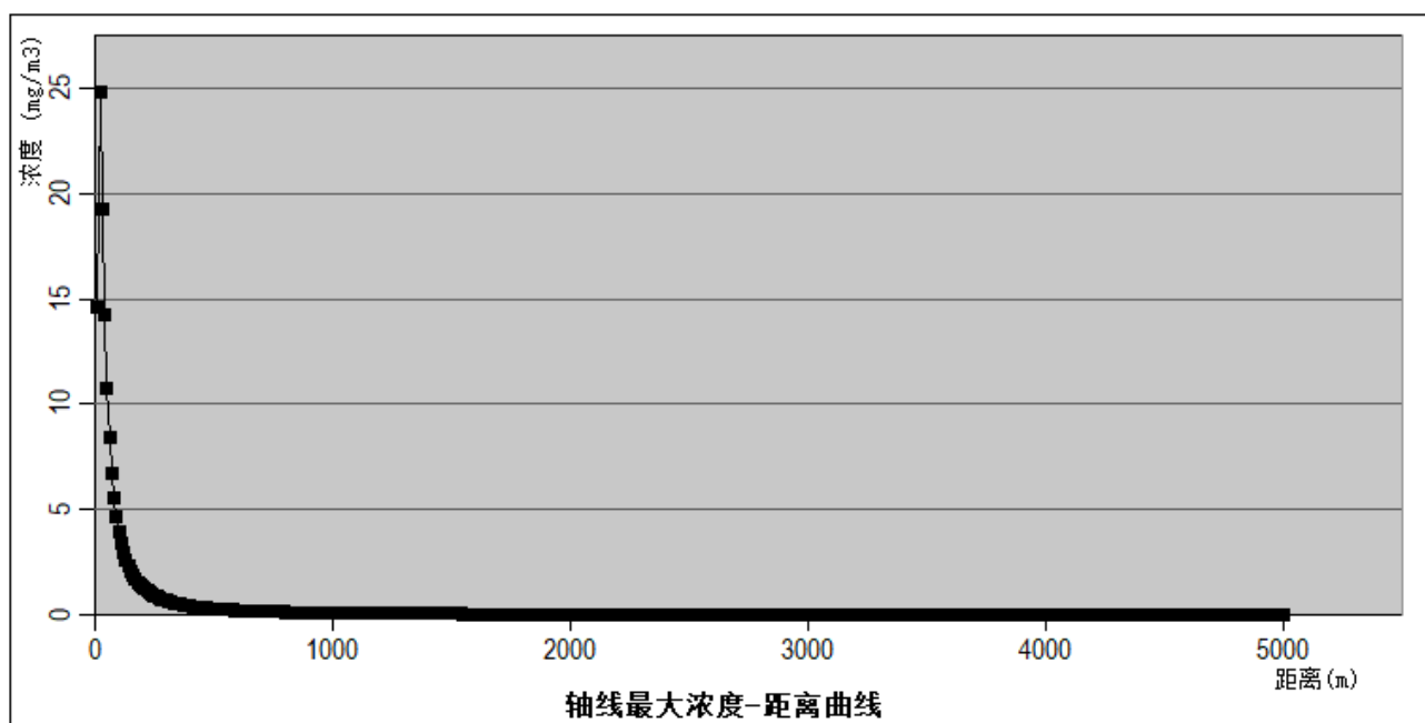
图6.8-7 最不利气象条件下***泄漏最大浓度与距离关系图
