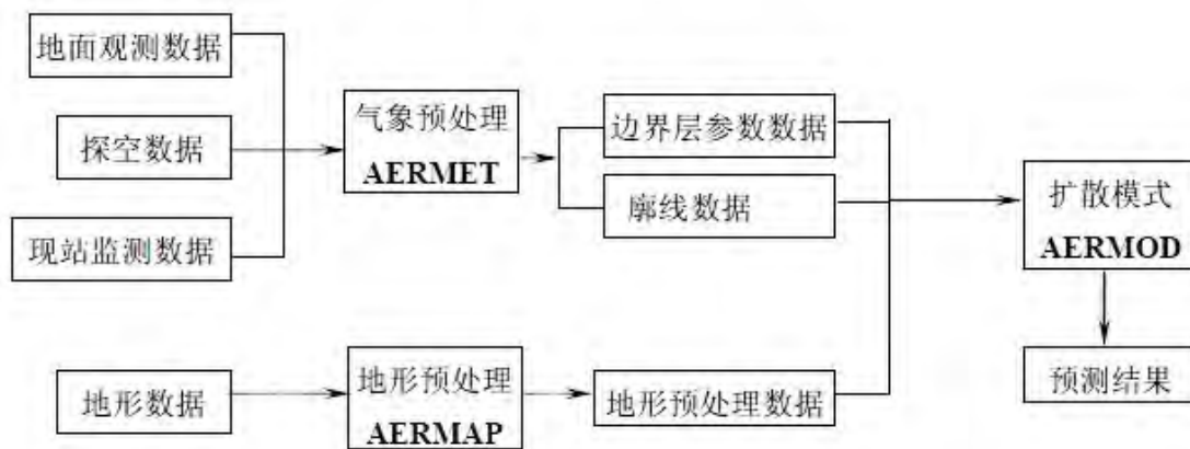
图6.2-10 AERMOD 模式系统流程图
