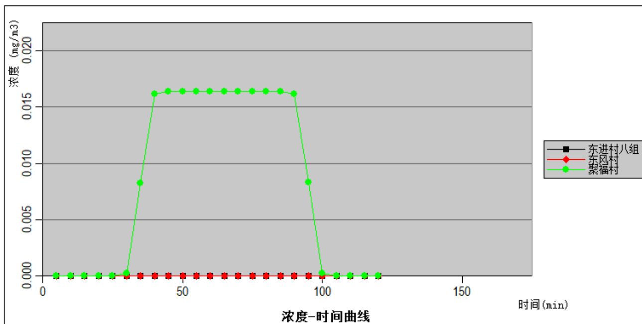
图6.8-20 氢氟酸（HF）泄漏各敏感点时间与浓度关系图（最不利气象）
