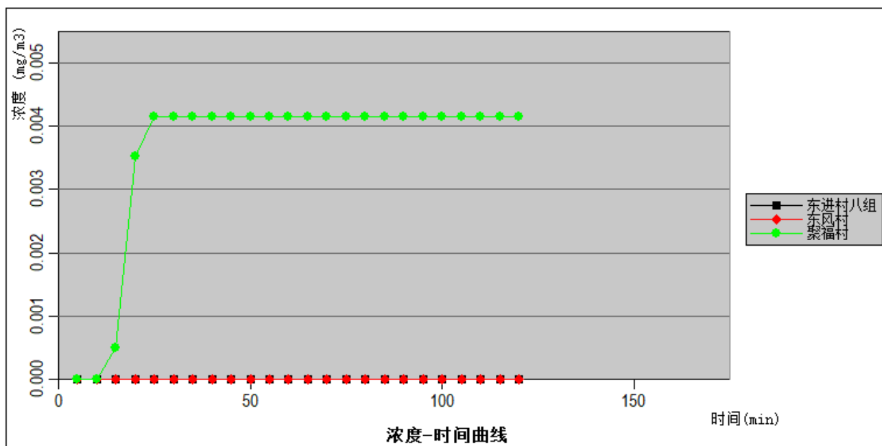
图6.8-9 ***泄漏各敏感点时间与浓度关系图（最不利气象）
