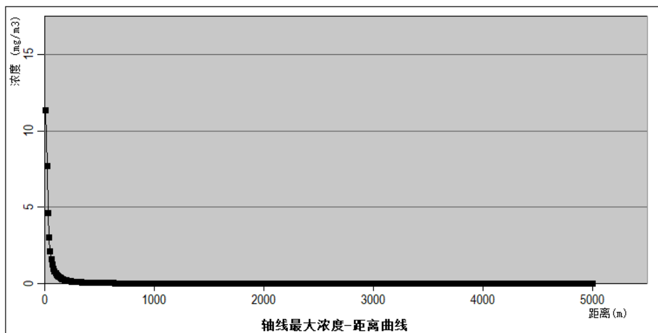
图6.8-18 最不利气象条件下氢氟酸（HF）泄漏最大浓度与距离关系图
