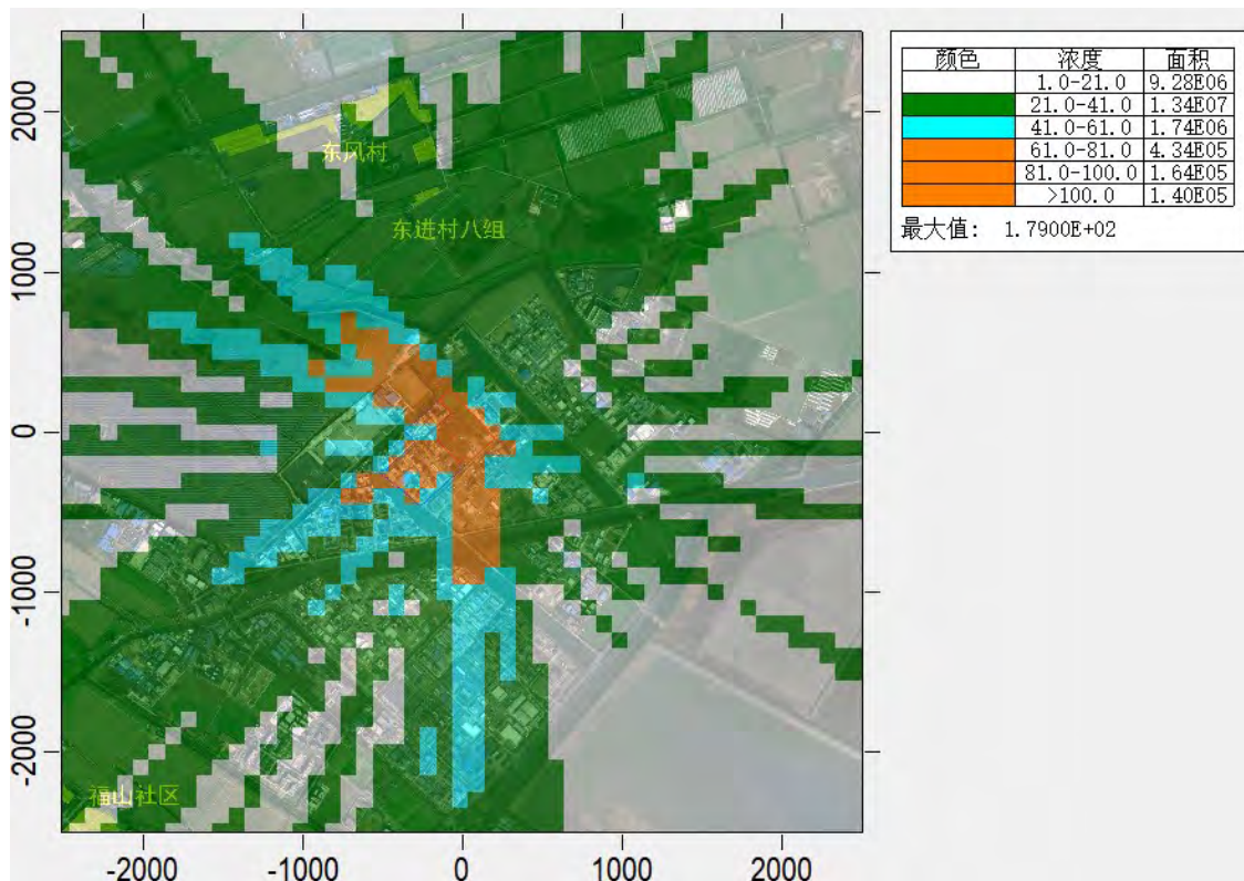
图6.2-25 非甲烷总烃 1 小时平均质量浓度贡献分布图（单位： \mu\text{g}/\text{m}^3 ）
