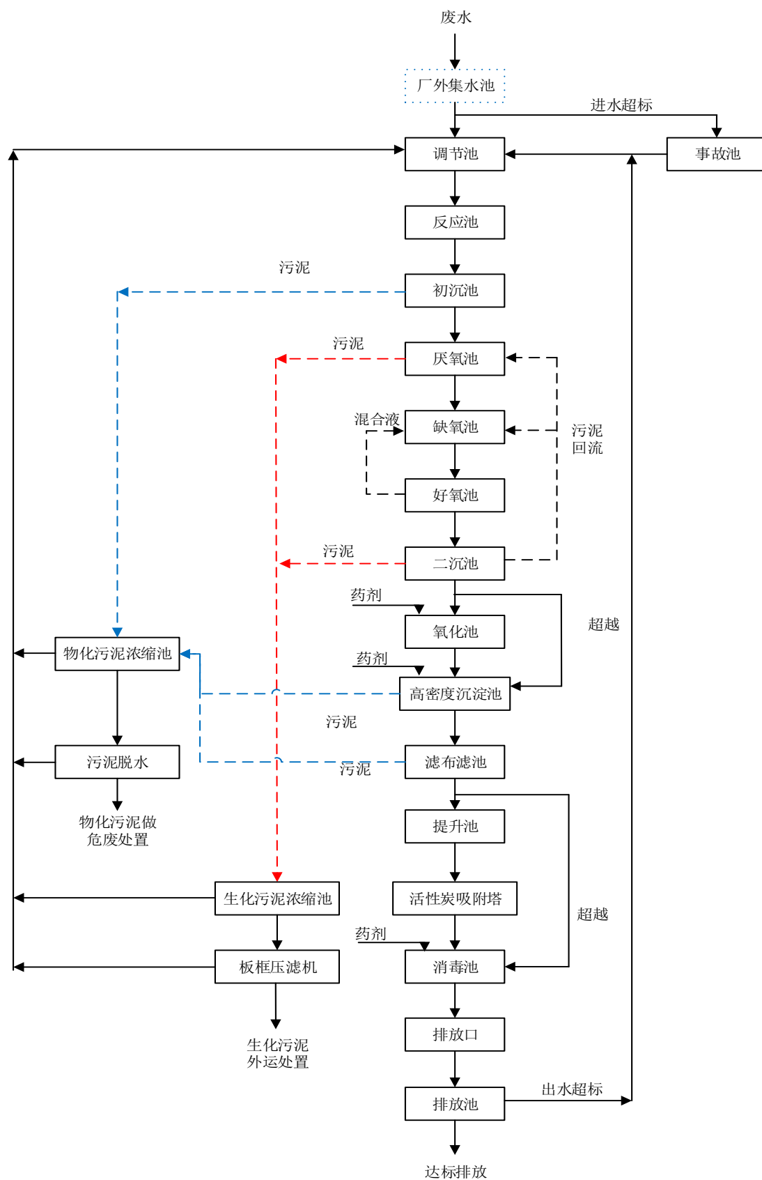
图7.2-2 常熟中法工业水处理有限公司工艺流程图
