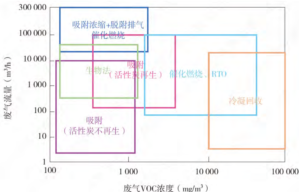
图7.1-2 VOCs 治理技术适用范围
