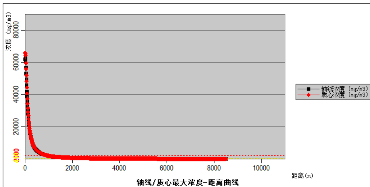
图6.8-4 最常见气象条件下 CTFE 泄漏最大浓度与距离关系图
