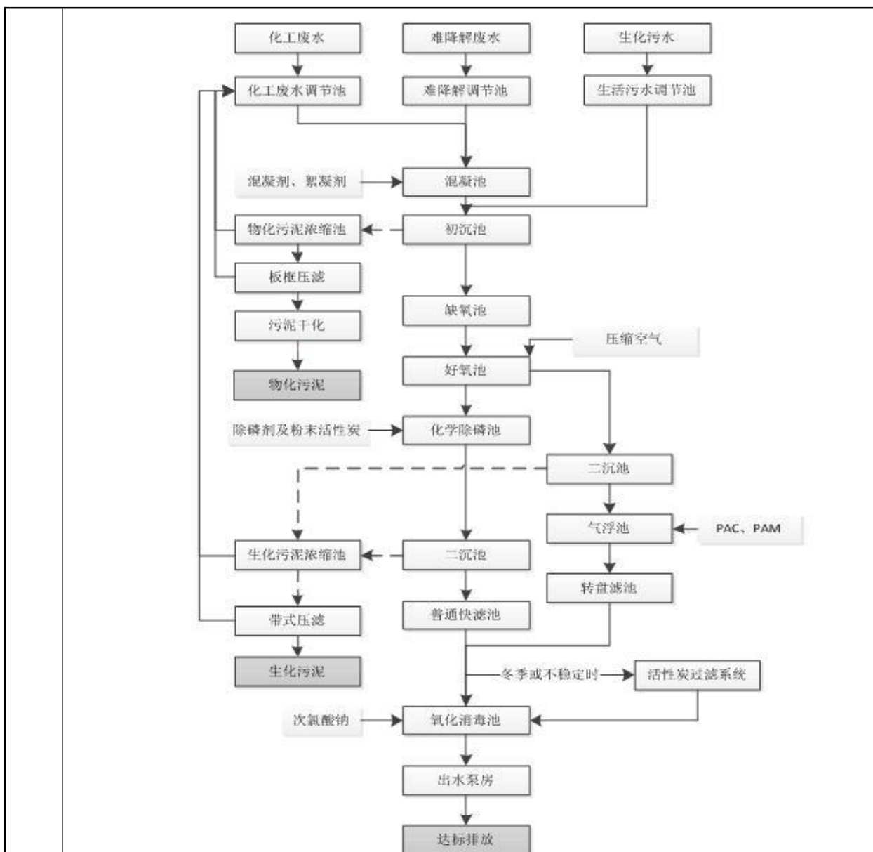
图 4-2 废水处理工艺流程图
