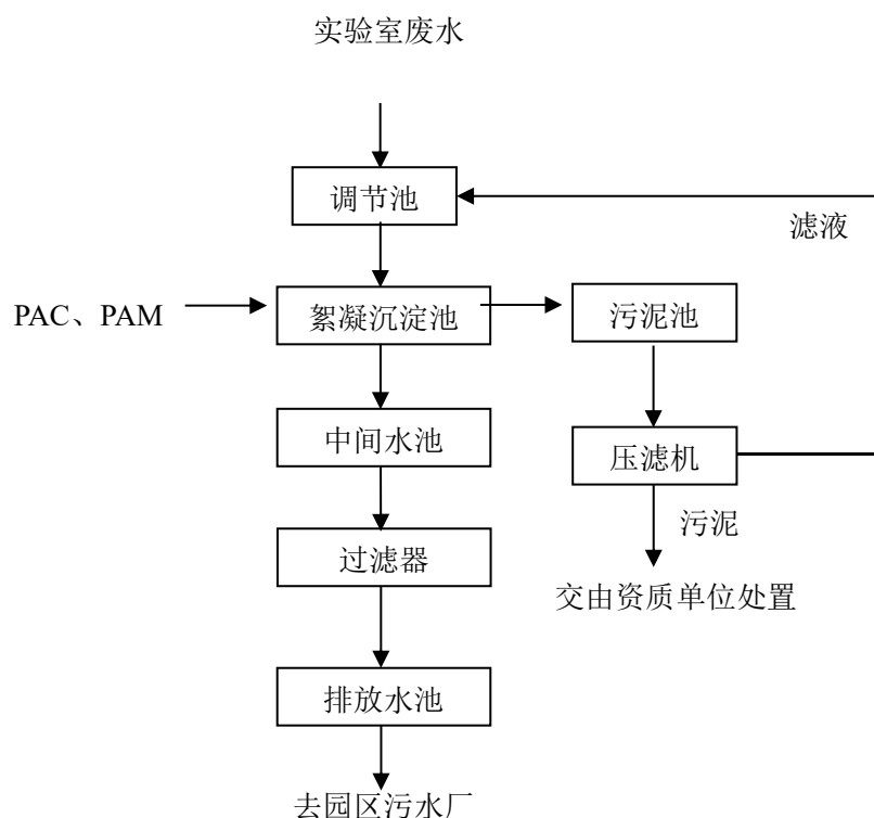
图 4-1 本项目污水处理工艺流程图
