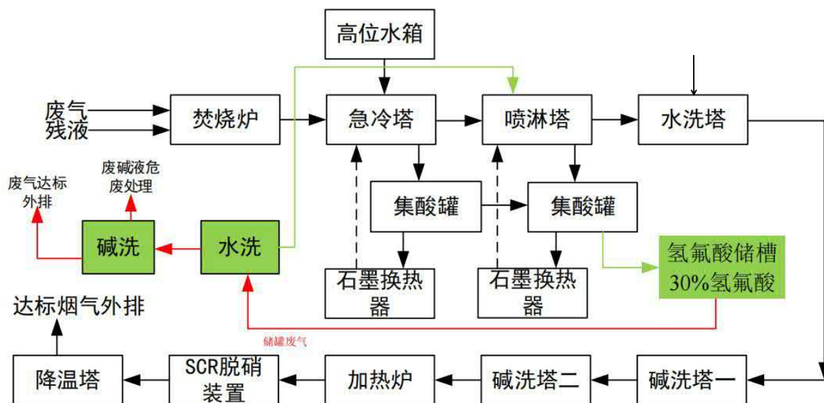
图 3.6.1-1 南厂区焚烧装置工艺流程框图
