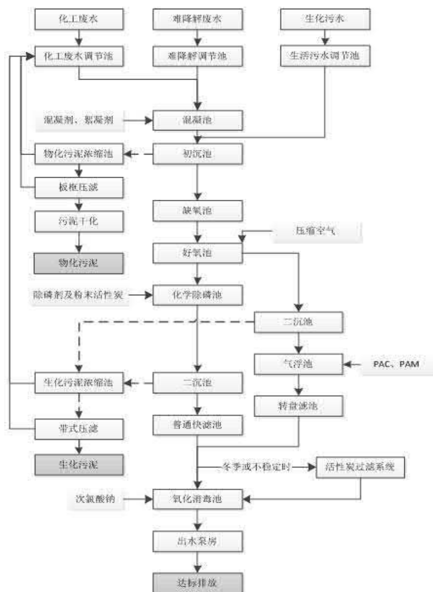
图 7.2-3 废水处理工艺流程图
