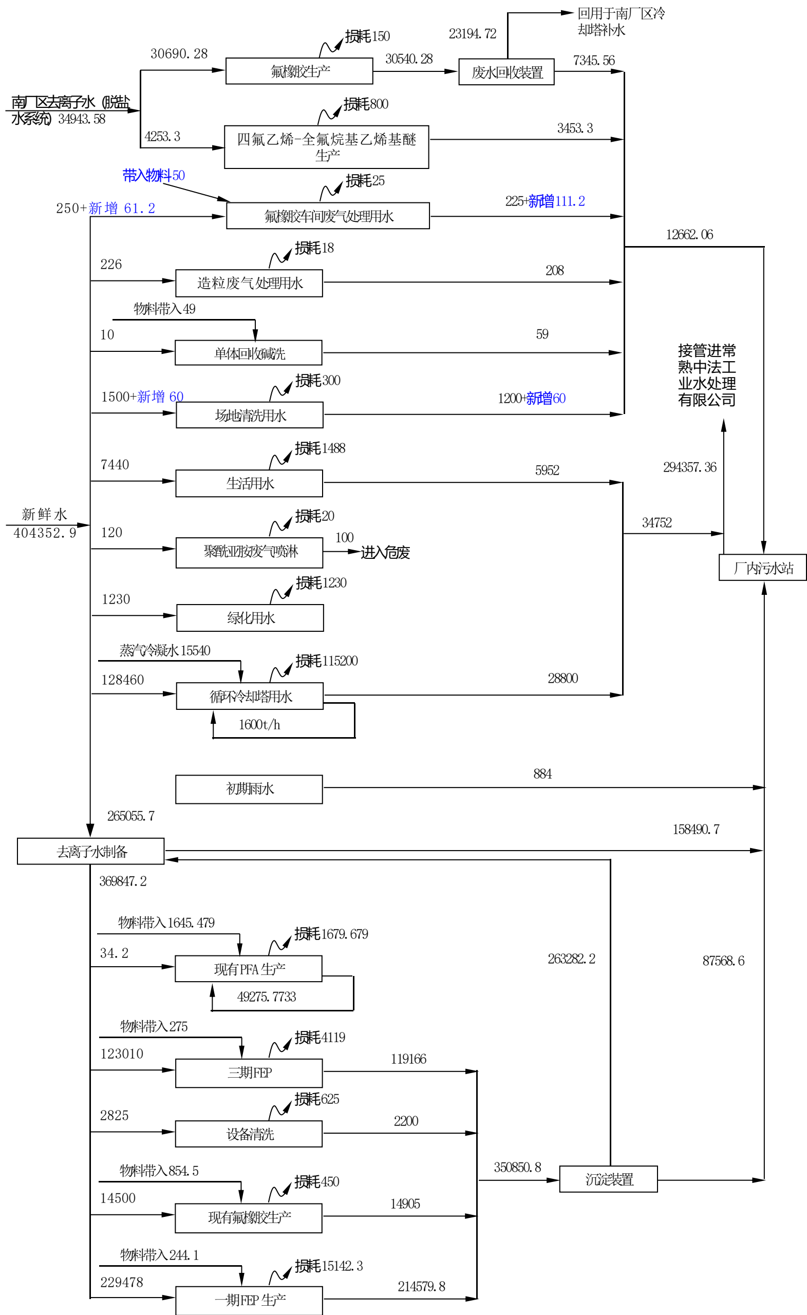
图 4.7-2 本项目建成后全厂水平衡图(m³/a)
