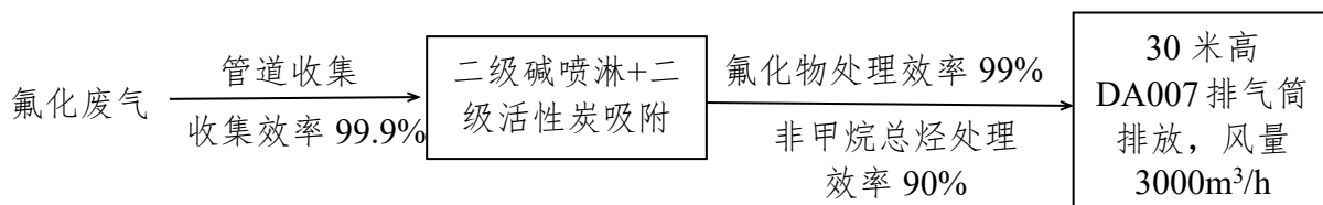
图 7.1.1-1 本项目废气处理工艺流程图
