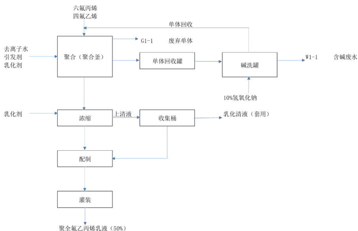
图 3.4.1-1 聚全氟乙丙烯乳液生产工艺流程图
