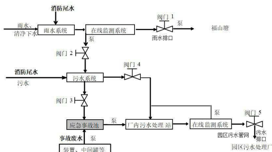
图 7.7.2-1 防止事故废水进入外环境的控制、封堵系统示意图
