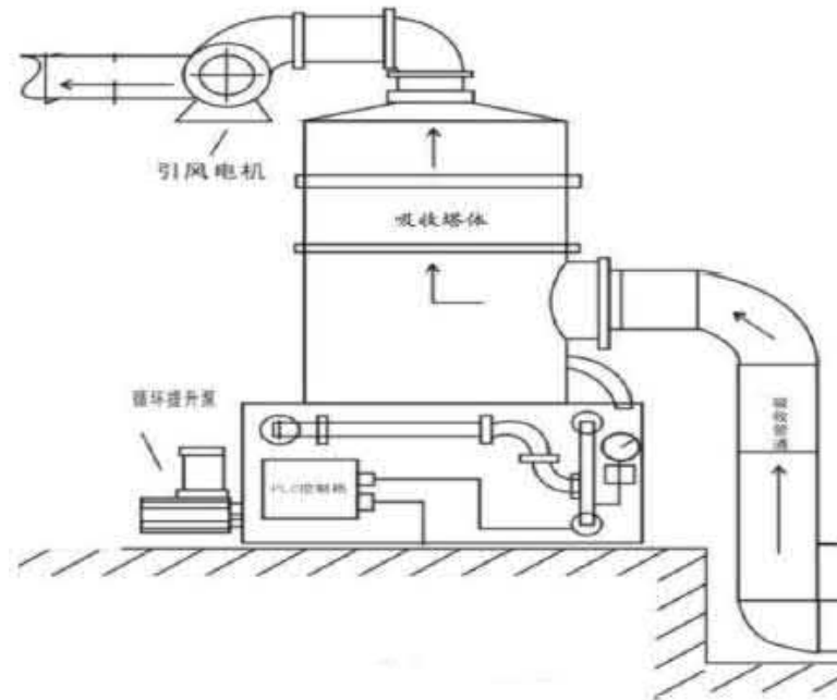
图 7.1.1-2 碱喷淋塔结构示意图
