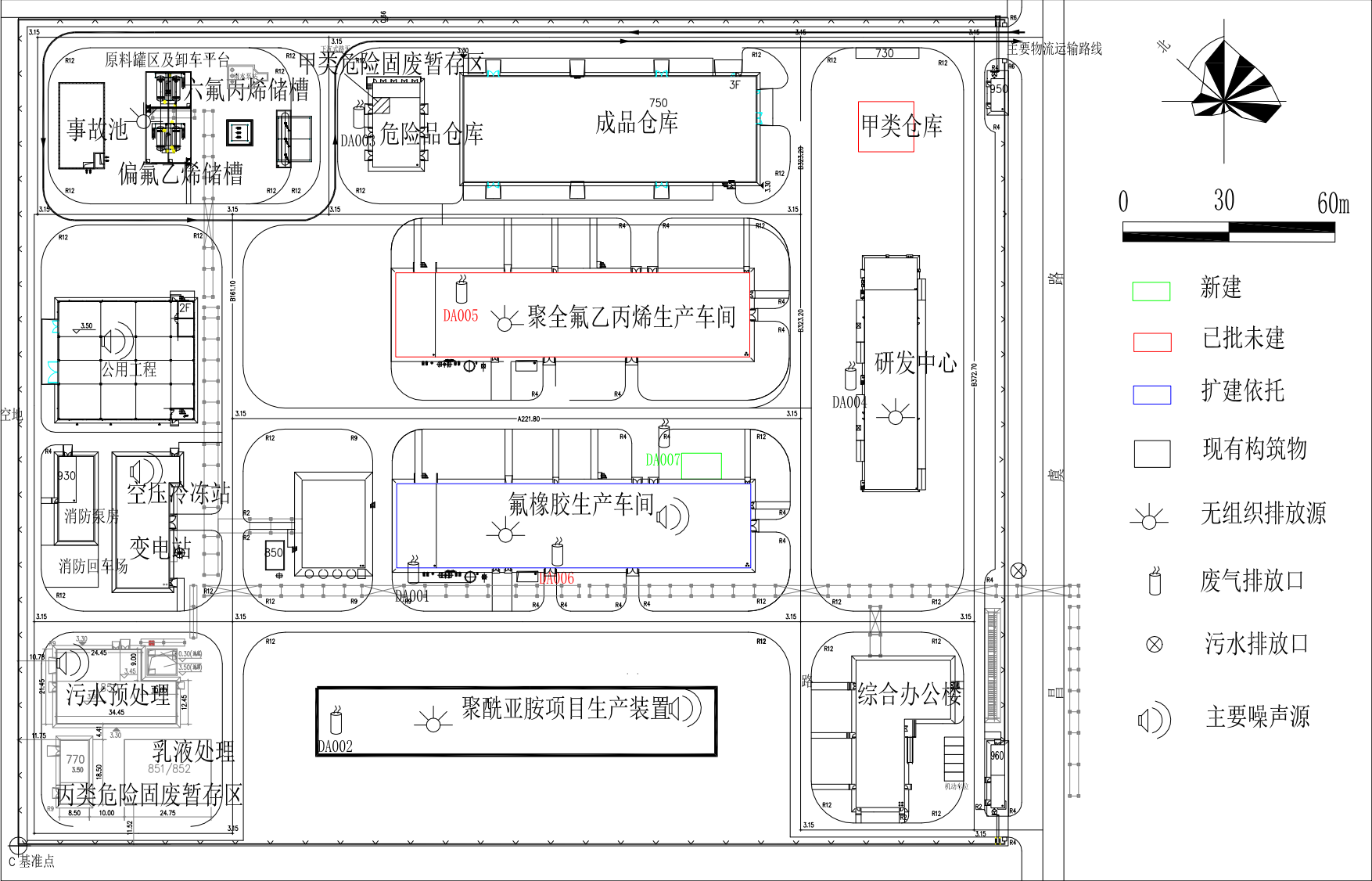
图 4.1.3-2 本项目改建后厂区平面布置图
