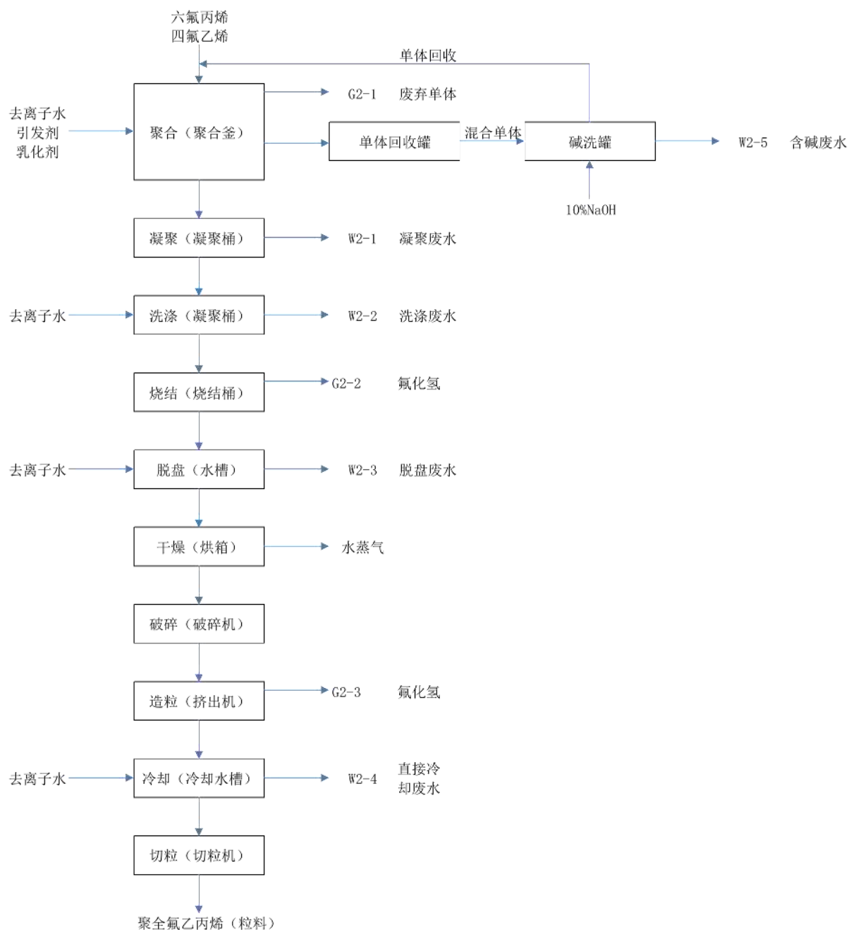
图 3.4.1-2 聚全氟乙丙烯（粒料）生产工艺流程图
