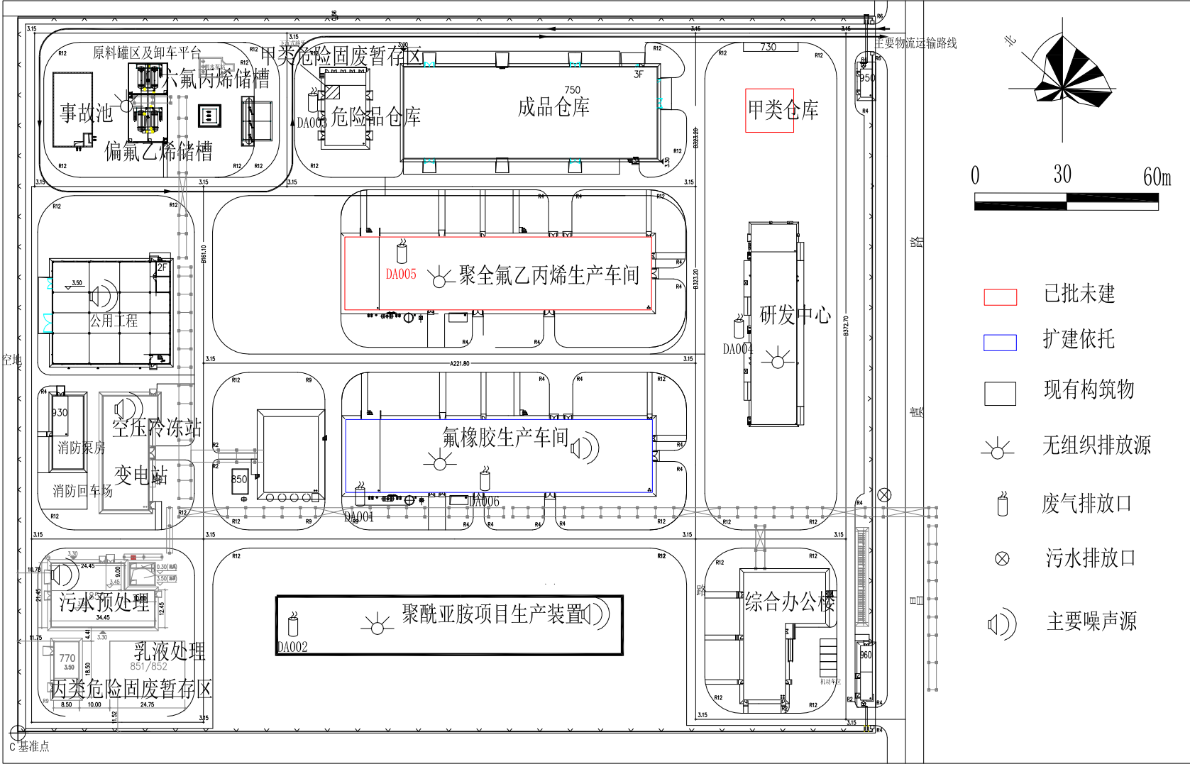
图 3.1-1 改建前北厂区现状平面布置图
