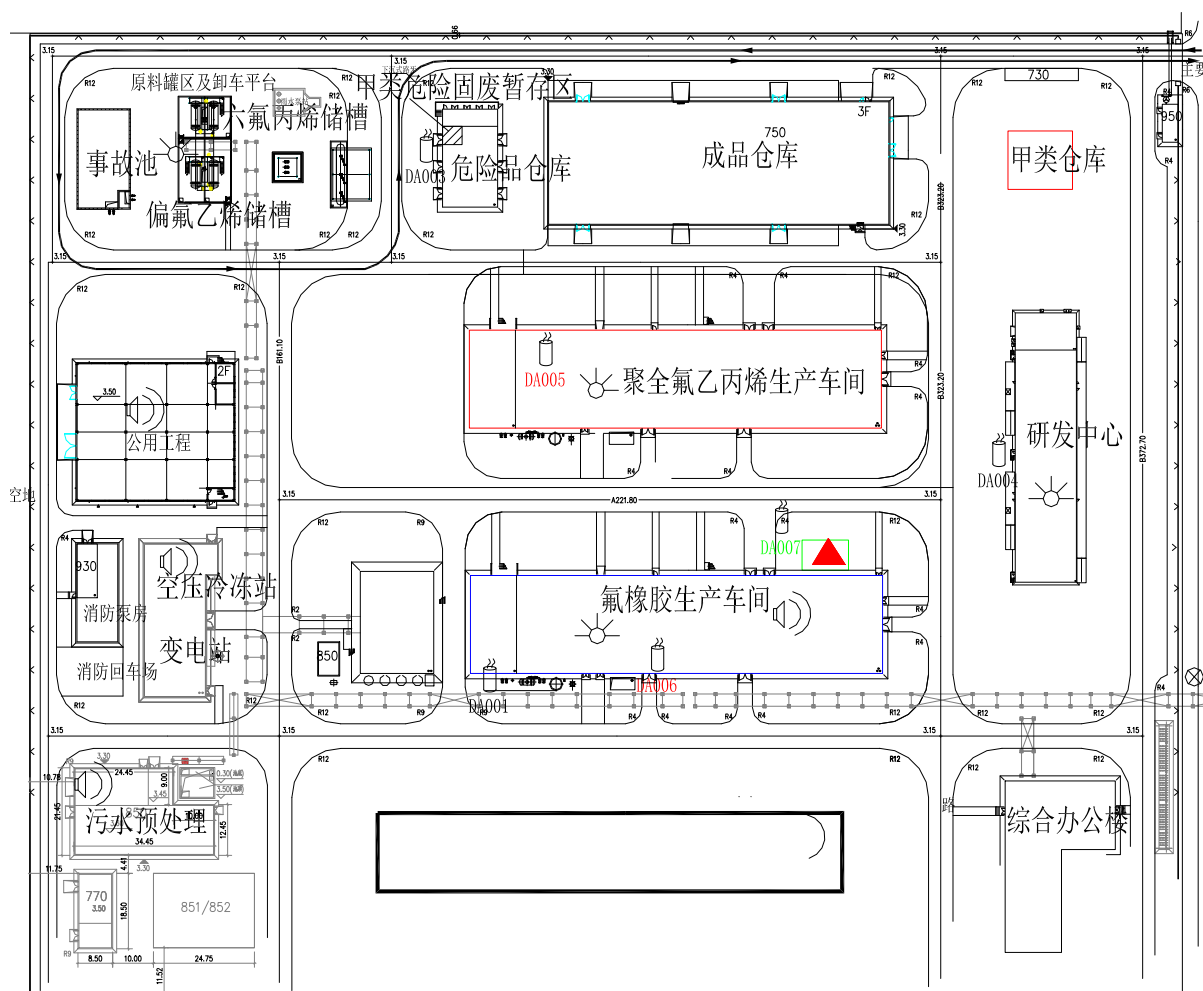
图 4.11.3-1 本项目危险单元分布图
