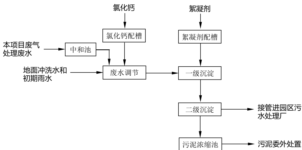
图 7.2-1 厂区污水站处理工艺流程
