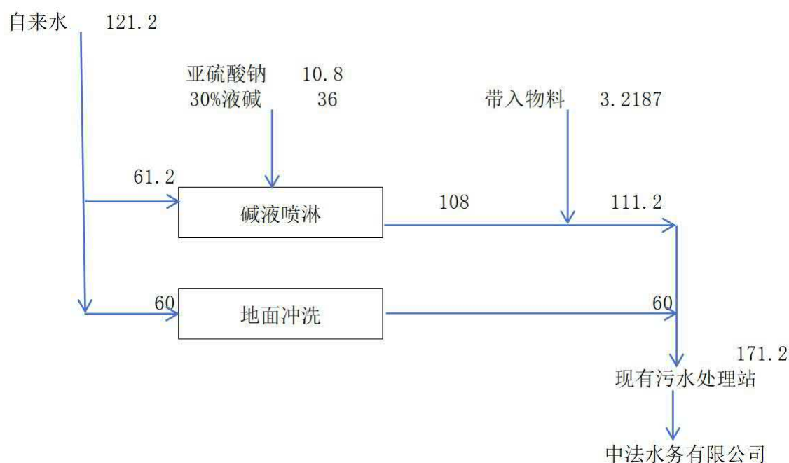
图 4.7-1 本项目水平衡图(m³/a)
