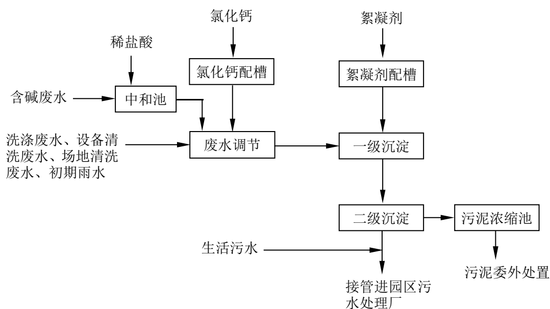
图 3.6.2-1 厂区污水站处理工艺流程
