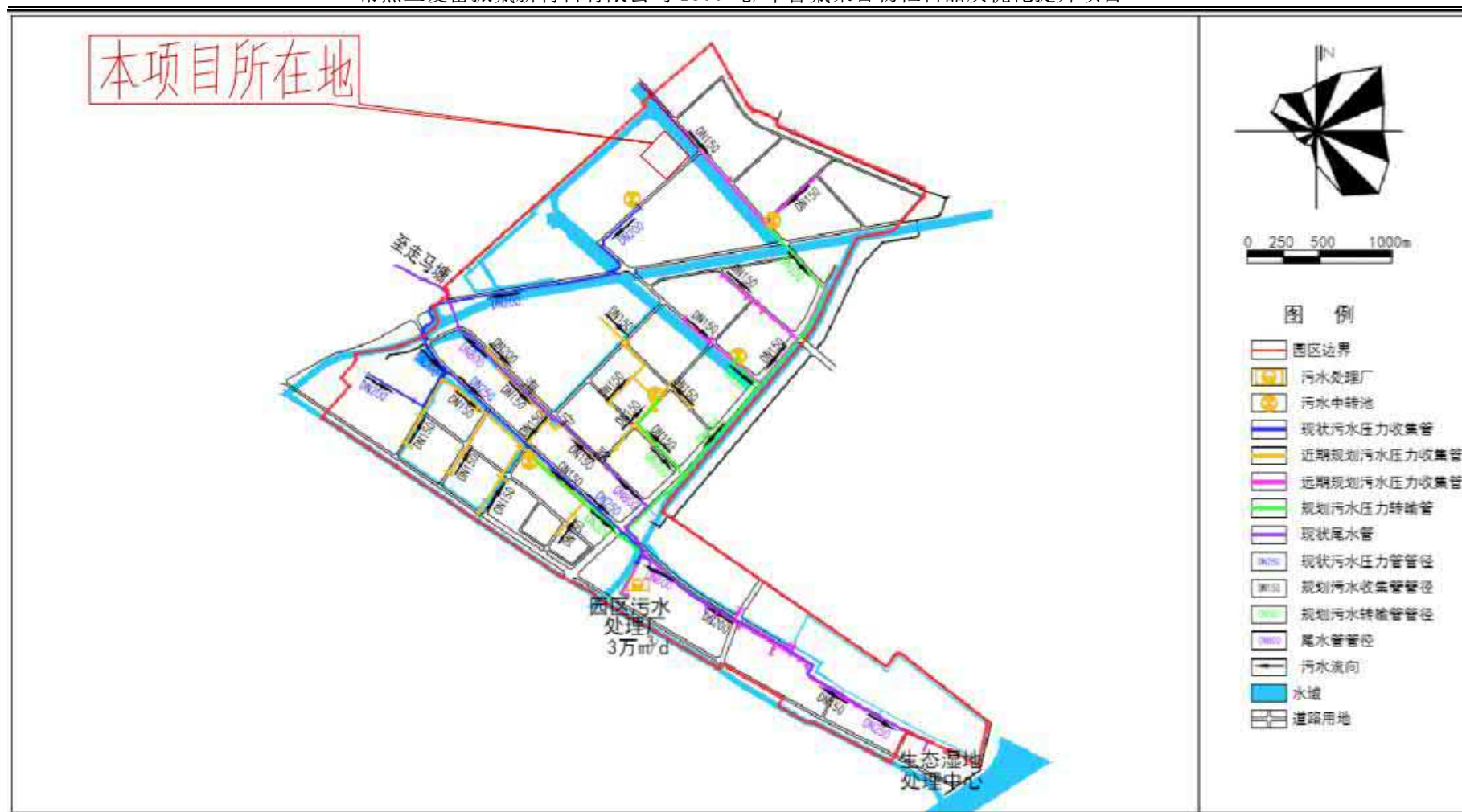
图 2.6.3-1 区域污水管网图
